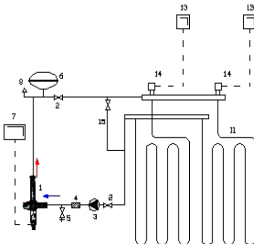
Схема подключения - обогрев пола
