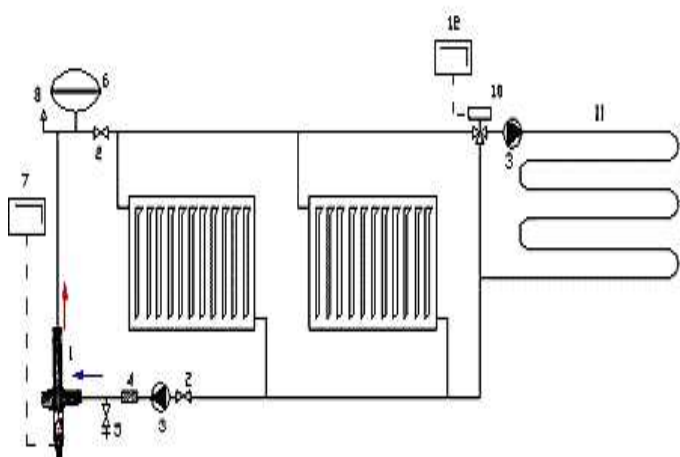
Схема подключения - радиатор + подогрев пола
