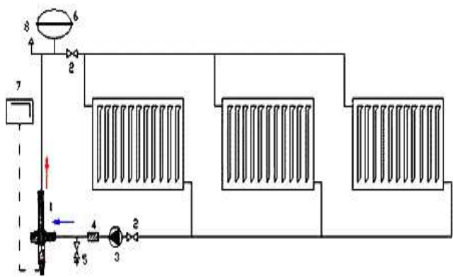
Схема стандартного подключения
